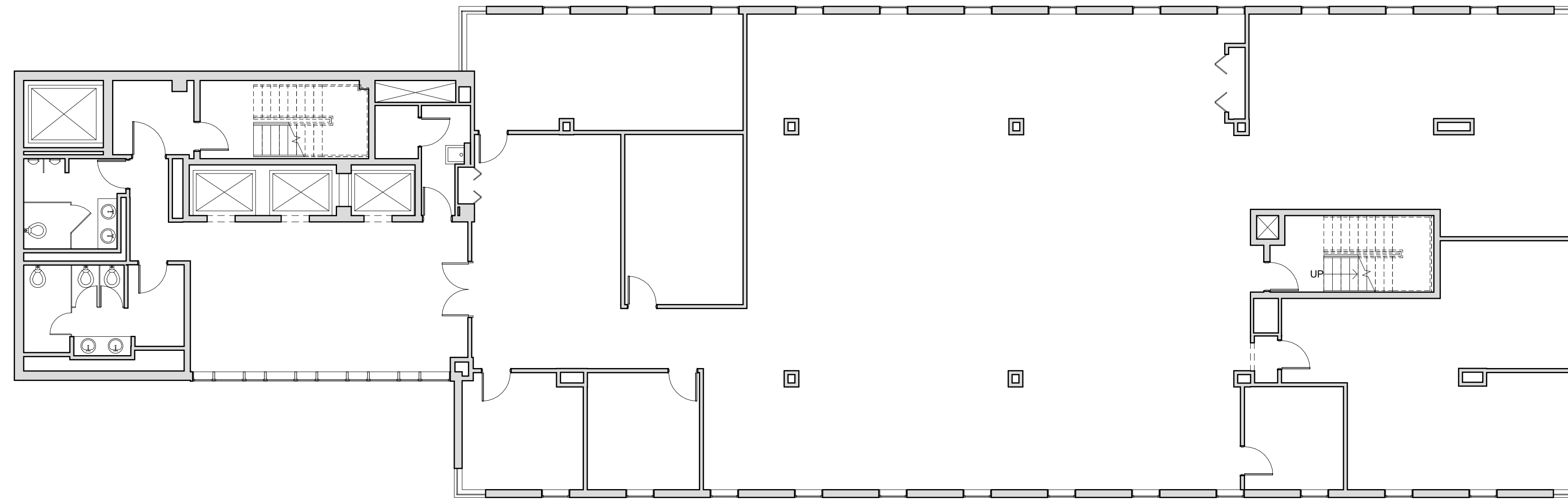
1 04 - FOURTH FLOOR SCALE: 1/8" = 1'-0"
